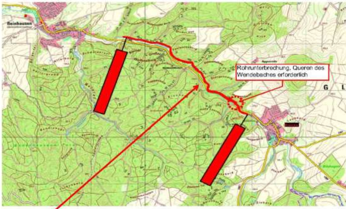
2 x Kabuflex Rohr DN 50 WD
